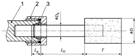
Bild 1: Einspannlänge von Spannflansch und Spannzanze
